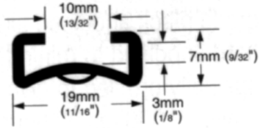
CALHA INOX
